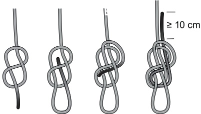
图1 八结图细节
